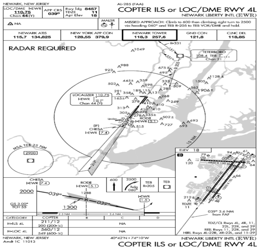
Figure 3-14. EWR Copter ILS Runway 4L
