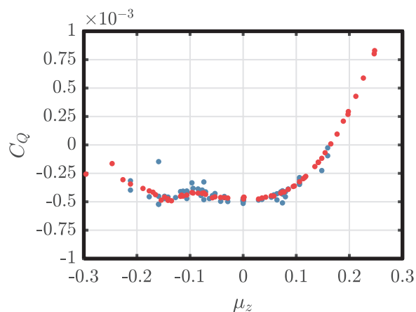
(d) upper rotor torque coefficients
