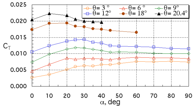
c) V/V_{tip} = 0.10
