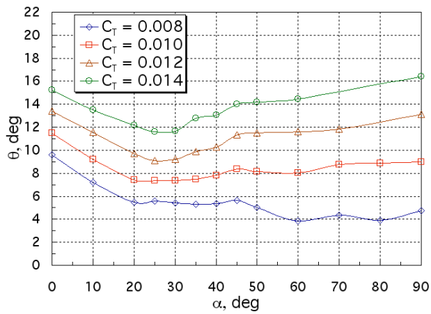
b) V/V_{tip} = 0.10
