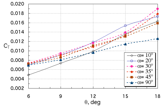
a) V/V_{tip} = 0.08
